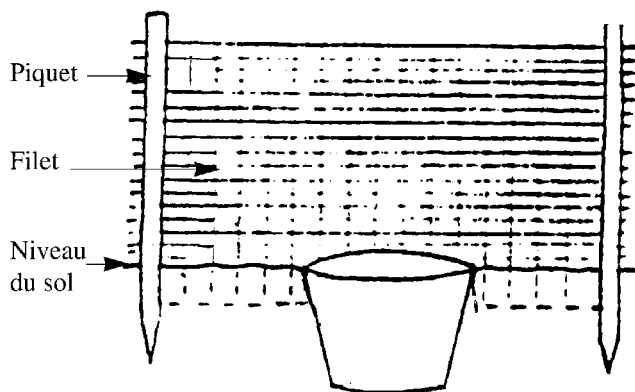
Fig. 2 : Dispositif de capture. Les animaux se heurtent au filet dont la base est enterrée et, en le longeant, tombent dans les seaux, eux-mêmes enterrés
