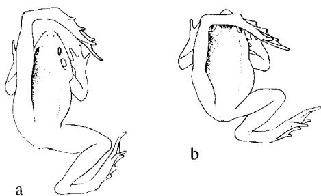
Fig. 4 : Un des caractères permettant de distinguer la Grenouille agile (a) de la Grenouille rousse (b) (Lanka & Vit 1985).
